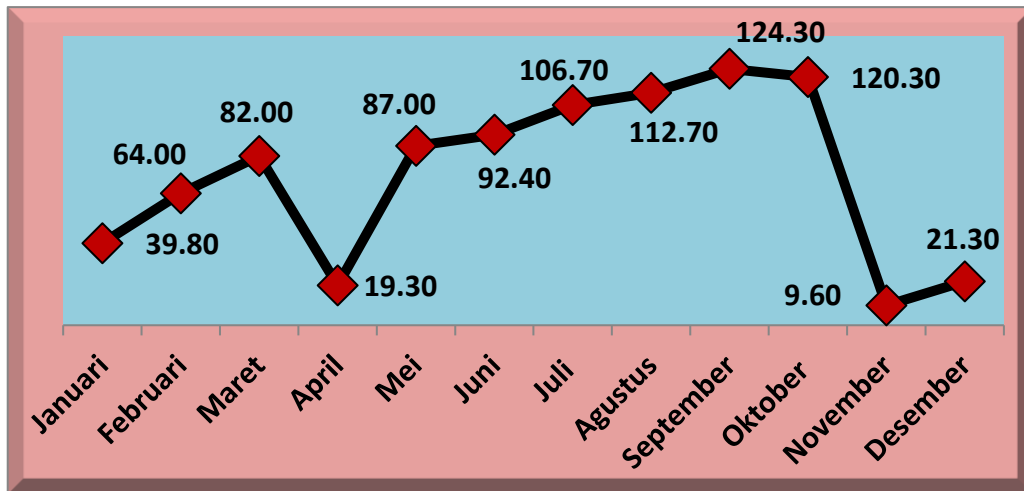
Gambar 2.3 Kondisi Curah Hujan di Kota Palu Menurut Bulan Tahun 2022
