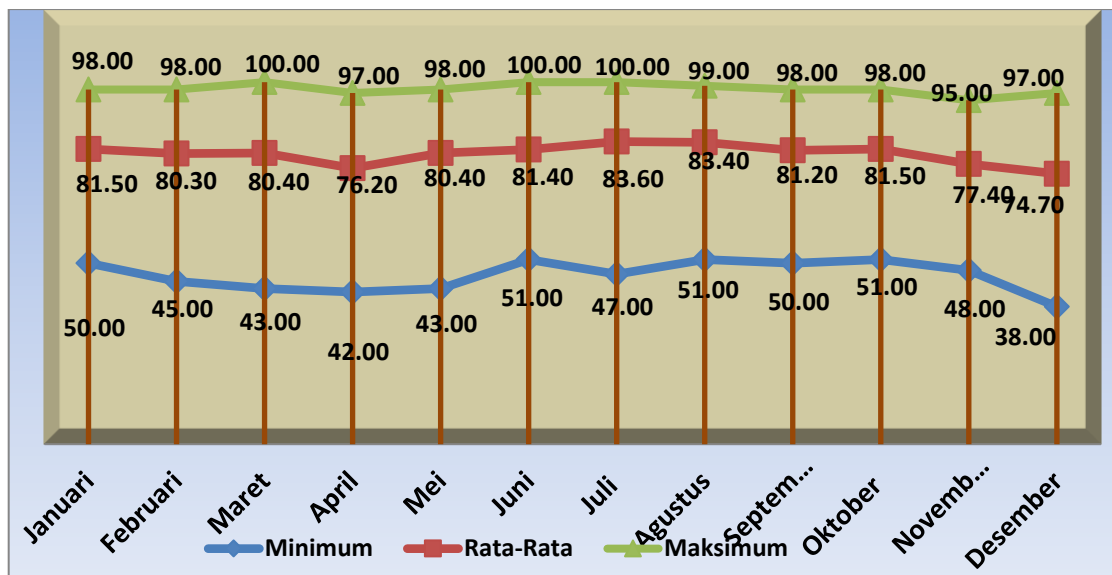
Gambar 2.4 Kelembaban Udara Minimum, Maksimum dan Rata-Rata Kota Palu Menurut Bulan Tahun 2022
