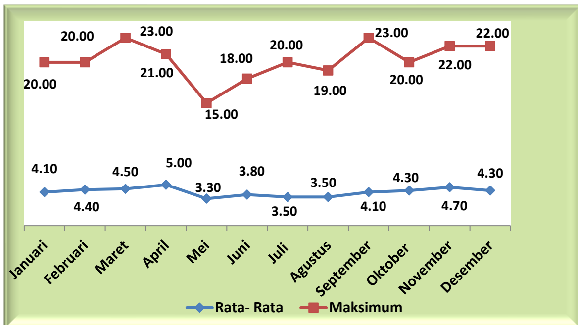
Gambar 2.5 Kecepatan Angin Kota Palu Menurut Bulan Tahun 2022
